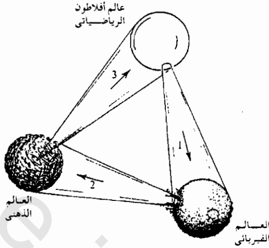
شكل (١-٣): ثلاثة عوالم: الفيزيائي والذهني والرياضي الأفلاطوني والعلاقات الغامضة بينهم.
