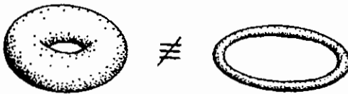
شكل (٨-١١): طارتان غير متكافئتين.
