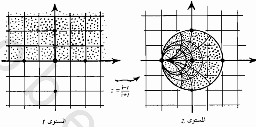
شكل (٨-٨): التناظر z = \frac{-t+i}{t+i} ، t = \frac{z-1}{iz+1} بدلالة المستويين المركبين t و z .
