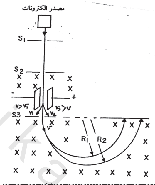
شكل (١-٥) مطياف الكتلة
