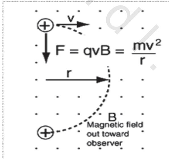
شكل (١-٦) تأثير المجال المغناطيسي علي الشحنة
