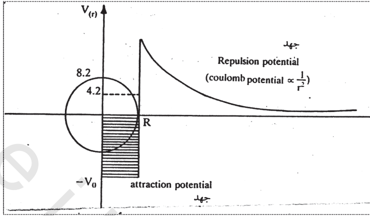
شكل (٤-٤) يوضح شكل الجهد النووي لجسيمات ألفا
