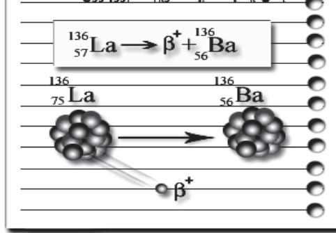
شكل (٤-٨) يوضح انحلال جسيمات بيتا الموجبة.
