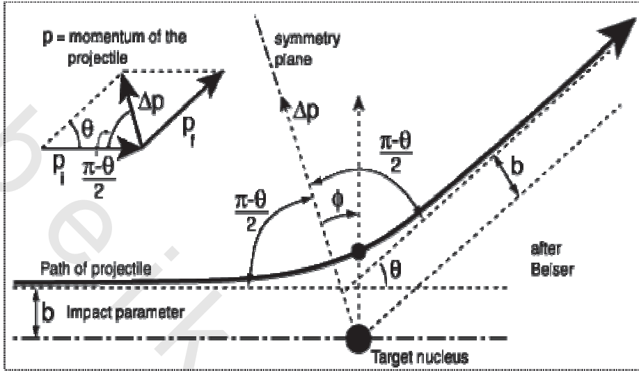
شكل (5-4) يوضح استطرارة رذرفورد
