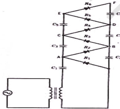
شكل (٧-١) معجل كوكورفت والتون
