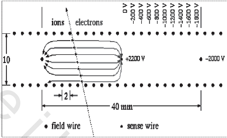
شكل (٨-٧) تركيب حجيرة التدفق
