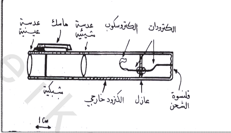
شكل (٨-١٠) الكاشف الجيبى
