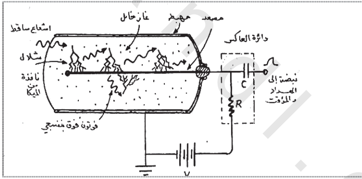
شكل (٨-٥) عداد جييجر - مولر
