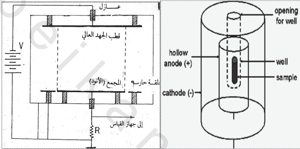
شكل (٨-١) غرفة التأين ذات قطبين مستويين
