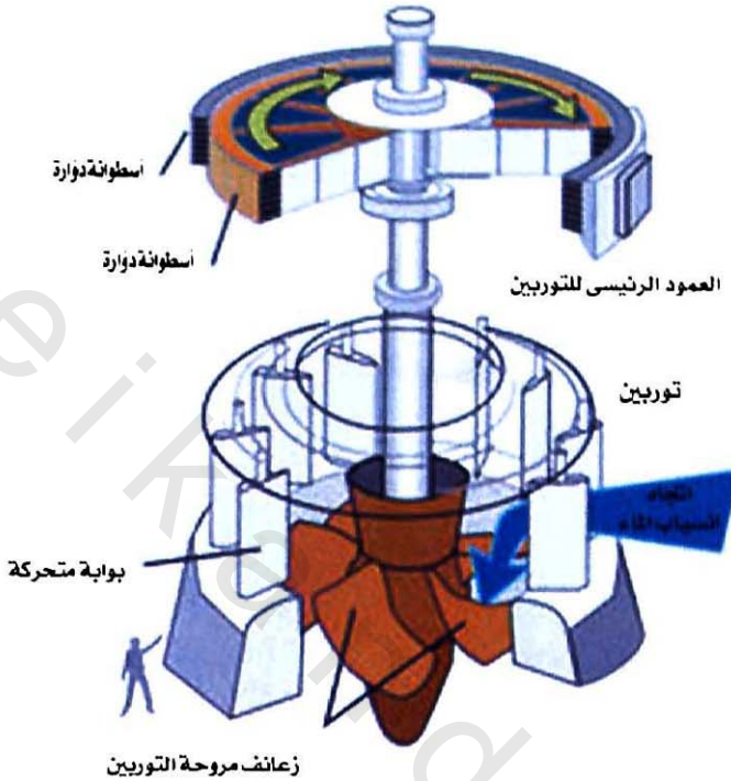
شكل (٨) : مقطع في توربين مائي
