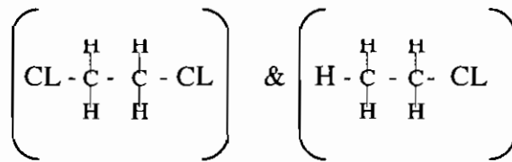
1,2 Dichloroethane
