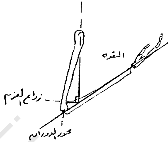
شكل ( ) ايضاح مكونات العزم في العمل العضلي
