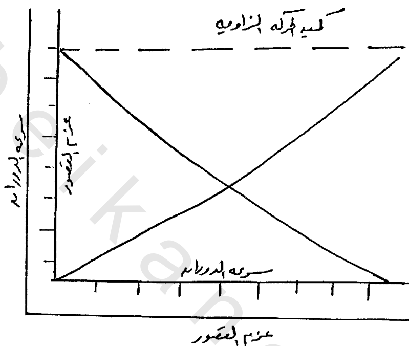
شكل ( ) علاقة عزم القصور الذاتي بالسرعة الزاوية خلال الطيران
