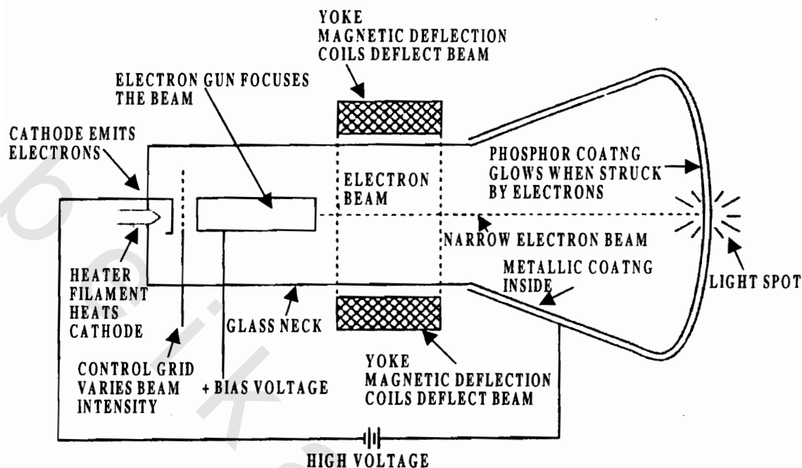
Fig. 12.17 CRT
