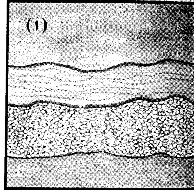
بعد أن ترسبت المواد العصرية في قاع البحار والمحيطات ، ومع حدوث تحركات أرضية تكونت طبقة من البترول بين الطبقات الصخرية بفعل الضغط أو الحرارة
