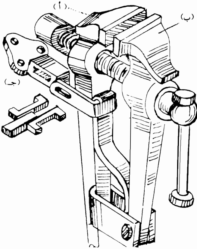
المنجلة الحدادی
