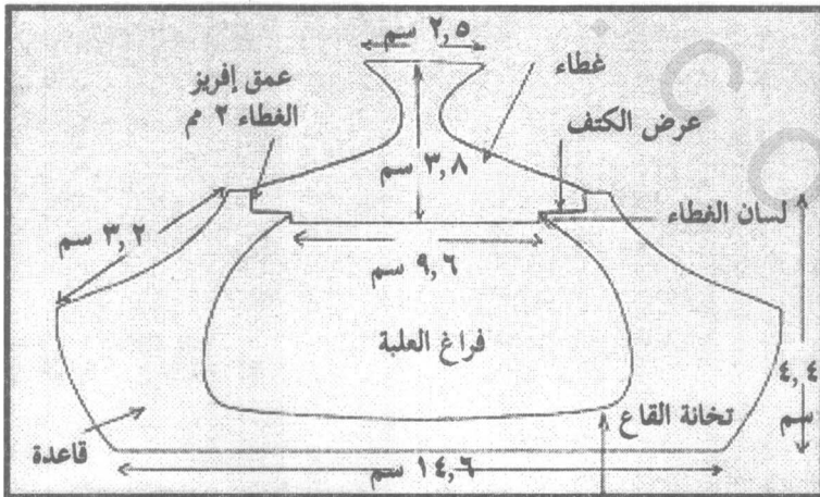
(شكل ٢-١٢) القاعدة والغطاء
