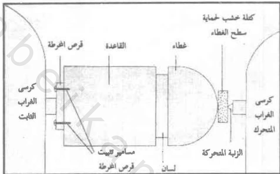
(شكل ٢-١٩) العلبه والغطاء على المخرطة
