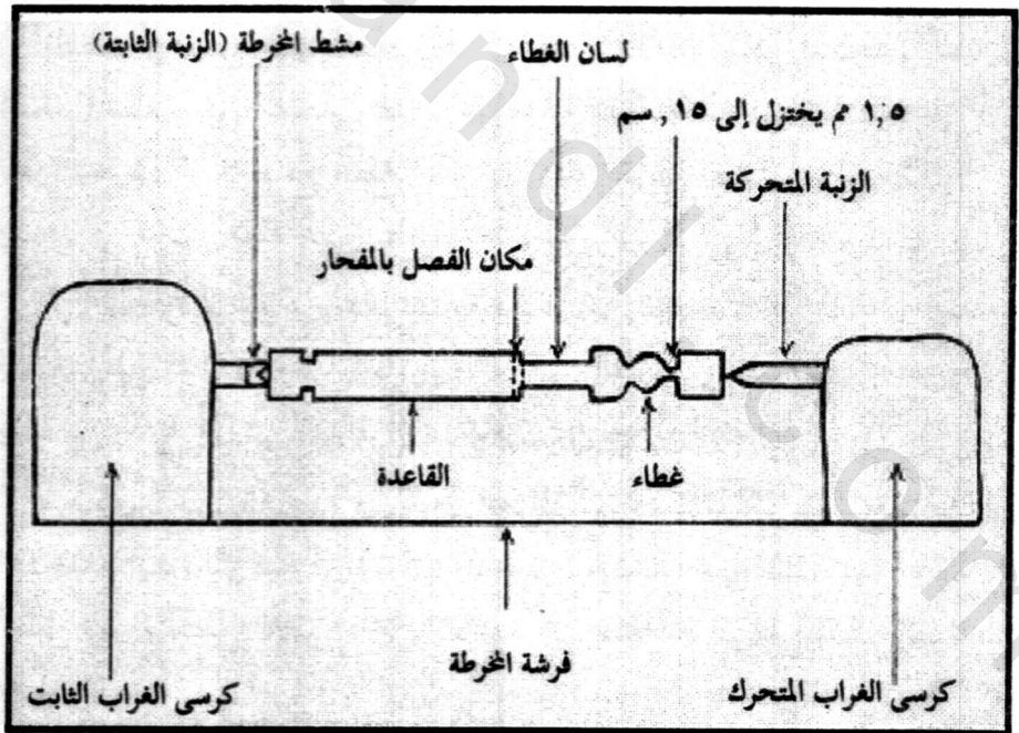
(شكل ٦-١٠) ويوضح فصل الفرز الغطاء (اللسان) من جهة القاعدة
