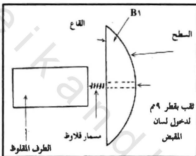
(شكل ٥-١٣) كتلة الغطاء على الطرف المقلوظ
