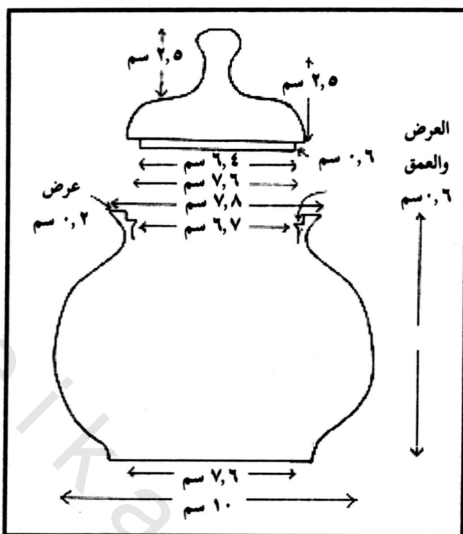
(شكل ١-٢) القاعدة والغطاء والمقاسات المختلفة لهما
