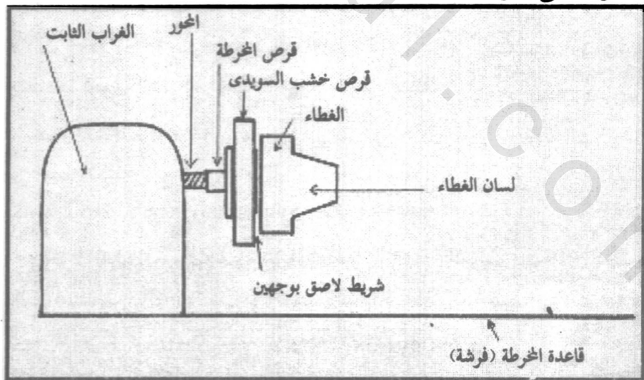
(شكل ٦-٢) يوضح برسم تفصيلى طريقة استعمال الشريط اللاصق ذى الوجهين مع قرص من خشب الموسيقى السويدى .. وكتلة الخشب.
