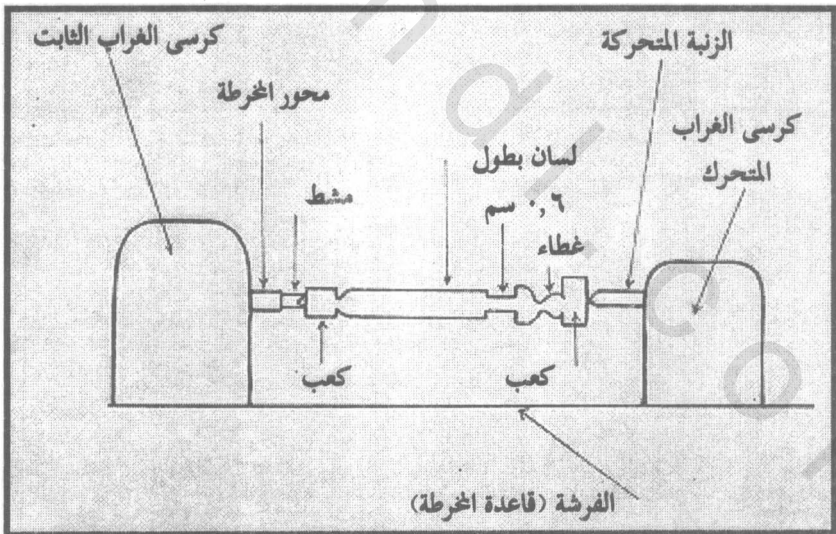
(شكل ٣ - ١٠) للعلبة والغطاء على محور واحد بين طرفي المخرطة ..
