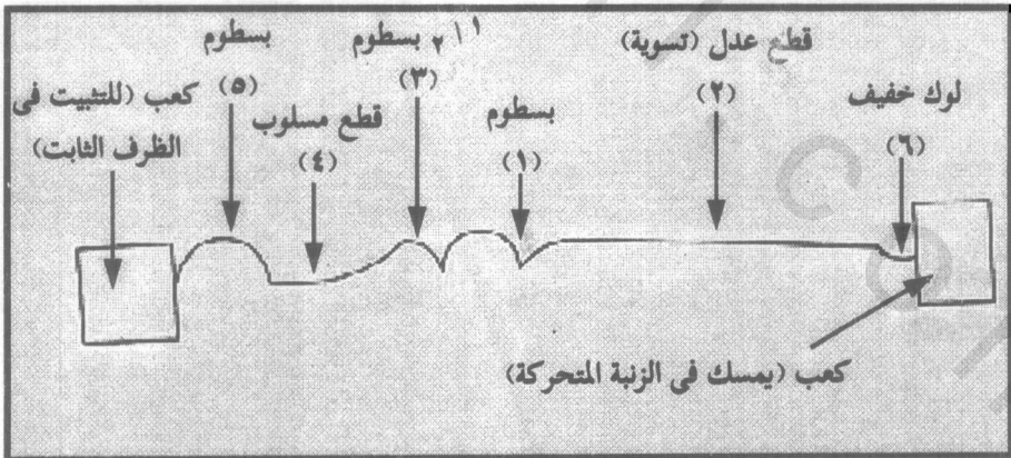
(شكل ٣-٢) بين الرسم التفصيلى لجراب القلم وشكل القطع والأدوات المستخدمة لتنفيذ كل شكل منها حسب الأرقام المكتوبة عليه
