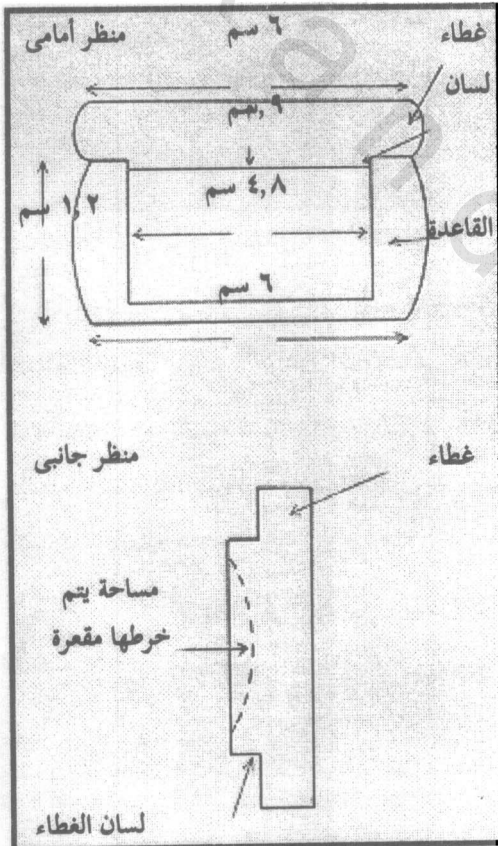
(شكل ٢-٧) القاعدة والغطاء
