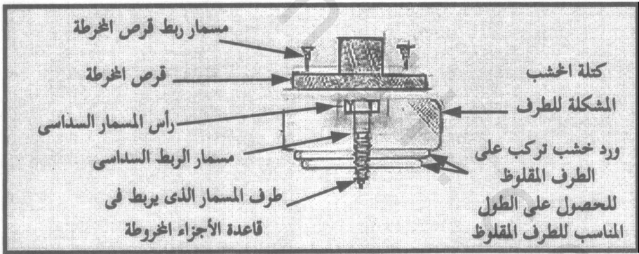
(شكل ١٠-١) رسم تخطيطى للطرف المقلوظ وطريقة تثبيته بقرص المخرطة
