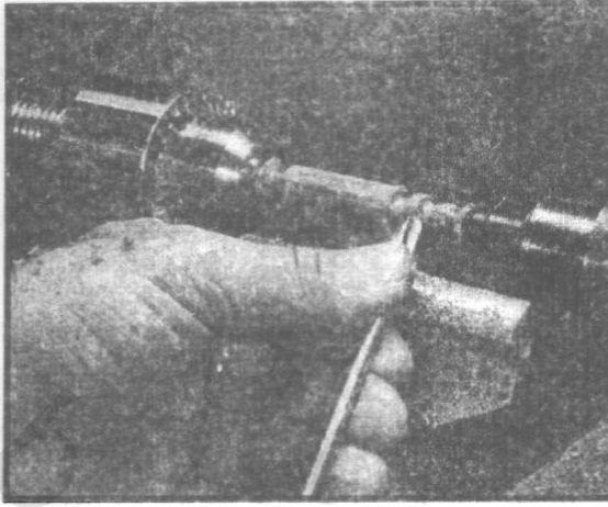
(شكل ٤ - ١٠) ويظهر طريقة خرط غطاء العلبة الأسطوانية الشكل بين طرفى المخرطة على محور واحد واستخدام الدفيرة لتشكيل خرط الغطاء من بسطوم ولوك ...
