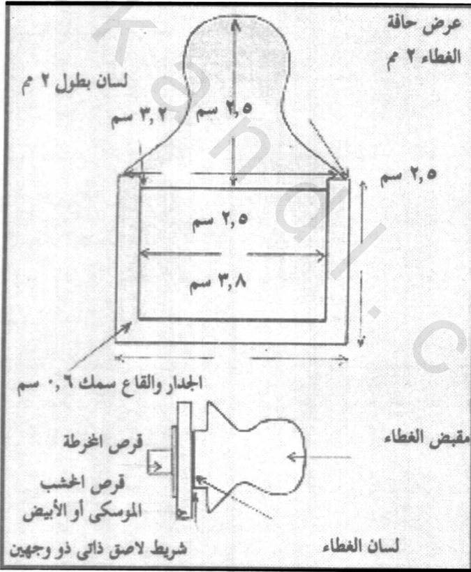
(شكل ٢-٩) علة صغيرة بالغطاء ( منظر أمامى وآخر جانبي )
