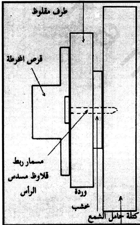
( شكل ٢-٥ ) طريقة تثبيت كتلة الخشب مع
