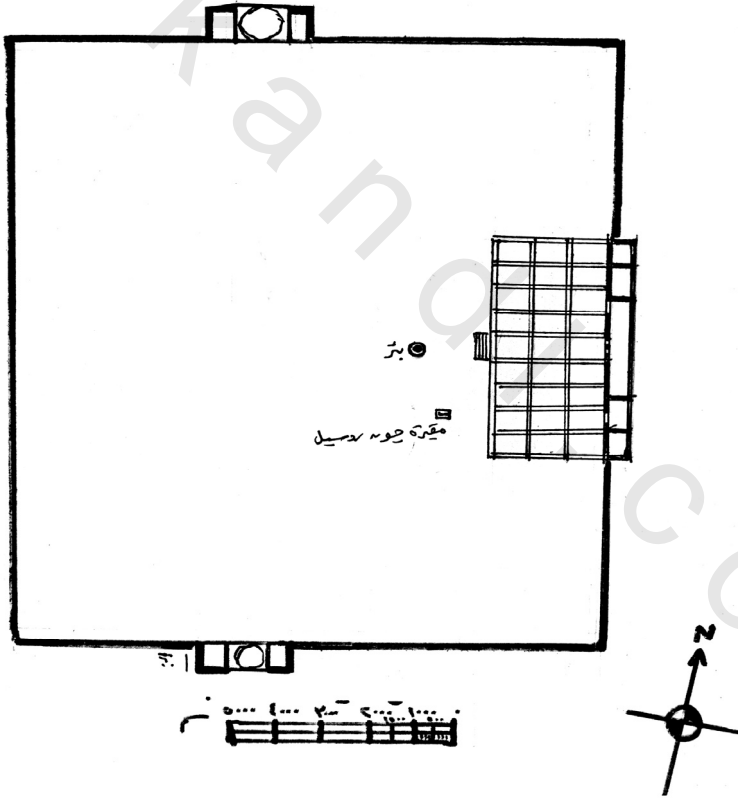
شكل (23) : مسقط أفقى لديوان العام بقلعة أجرا ، (من عمل المؤلف)
