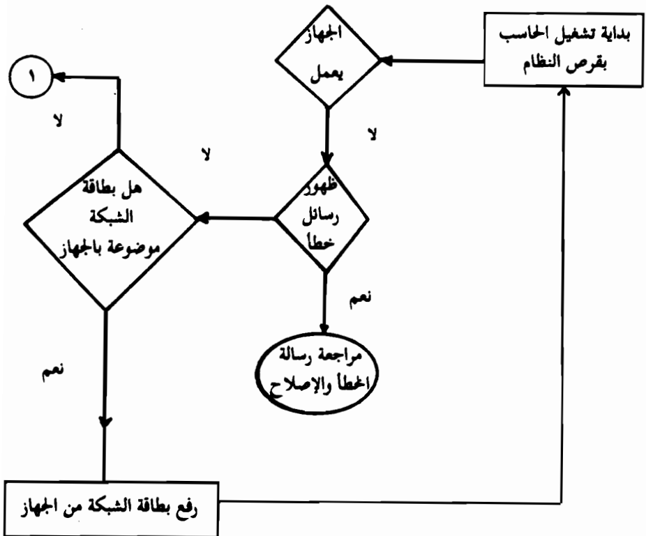
شكل (٤-٥) تتبع عطل فى شبكة نوفيل نتوير
