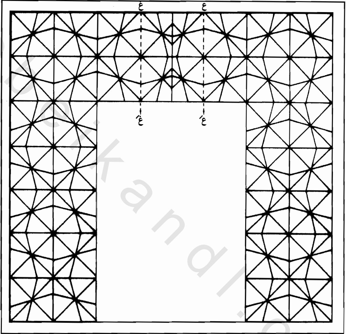
شكل (٧٢-١) الخطوط التأسيسية للشباك والذي استلّاع الفنان في العصر الإسلامي عن طريق الحذف والإضافة الحصول على الوحدات الرئيسية في التصميم الكلي العام كما في شكل (٦٩)
