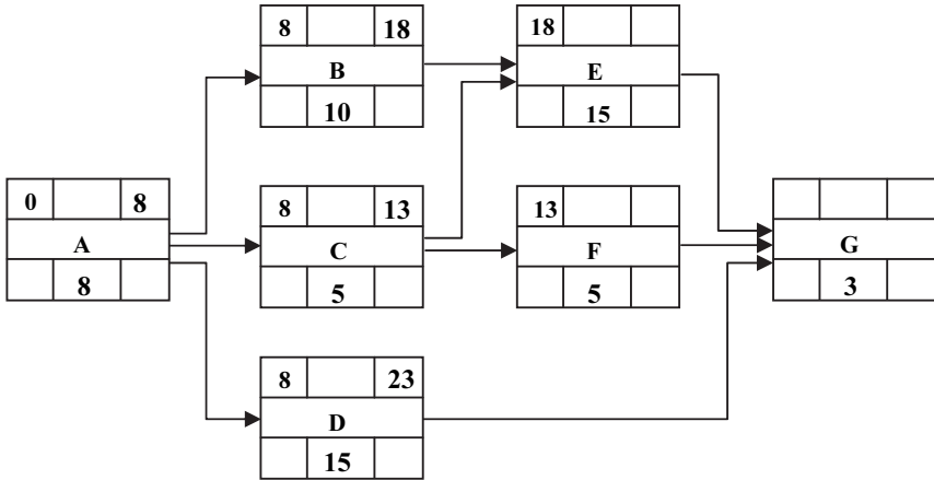
شكل (٣-٥١) حساب النهايات المبكرة للأنشطة (B&C&D) وتحديد البدايات المبكرة للأنشطة (E&F)
