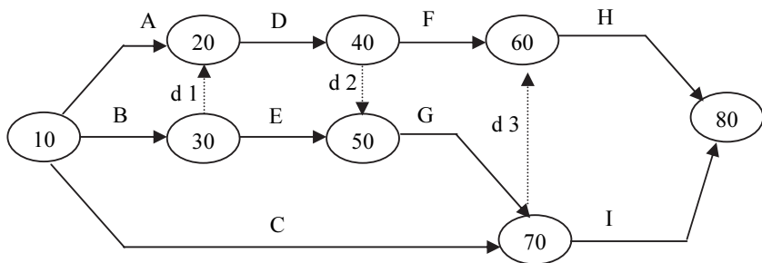
شكل (٤١-٣) رسم الشبكة بطريقة الأسهم
