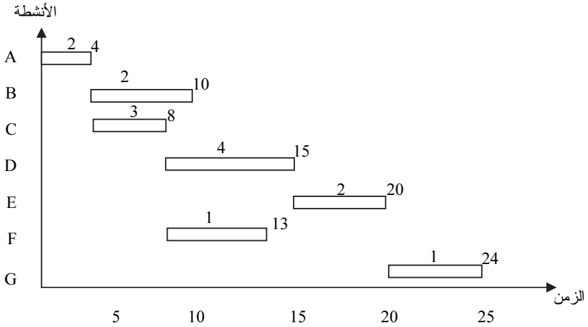
شكل (٧-٣) تمثيل البنود بطريقة الجدول البياني ويلاحظ أن زمن المشروع ٢٤ أسبوعاً
