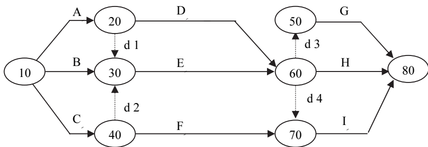
شكل (٣-٤٤) رسم الشبكة بطريقة الأسهم
