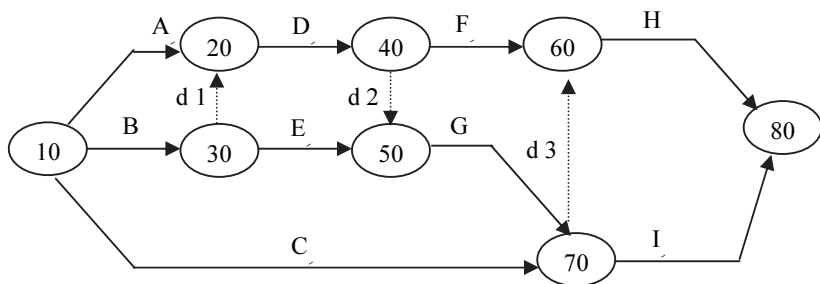
شكل (٣-٧٠) رسم الشبكة بطريقة الأسهم
