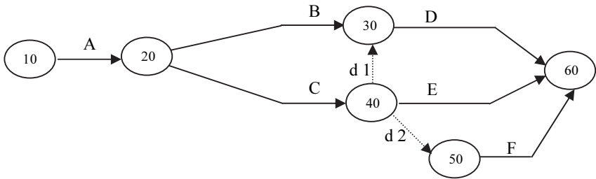
شكل (٣-٢٥) تجميع الأنشطة في نهاية المشروع
