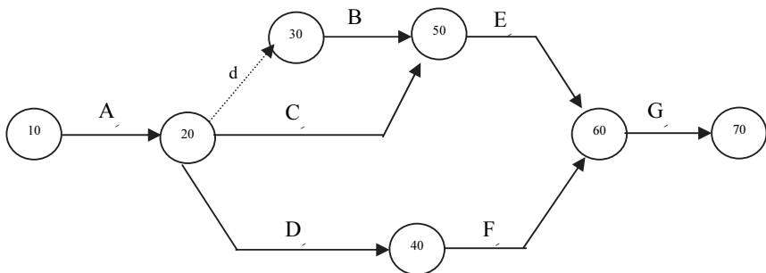
شكل (٣-٦٦) رسم الشبكة بطريقة الأسهم
