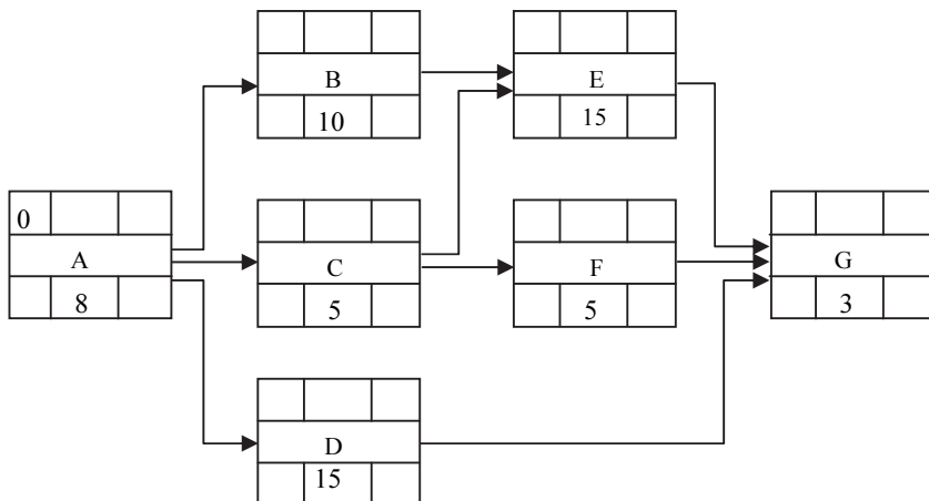
شكل (٣-٤٩) بداية الحسابات من زمن صفر كبدائية مبكرة للبند (A)
