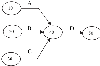
شكل (٣-١١) تمثيل مجموعة من الأنشطة بطريقة الأسهم
