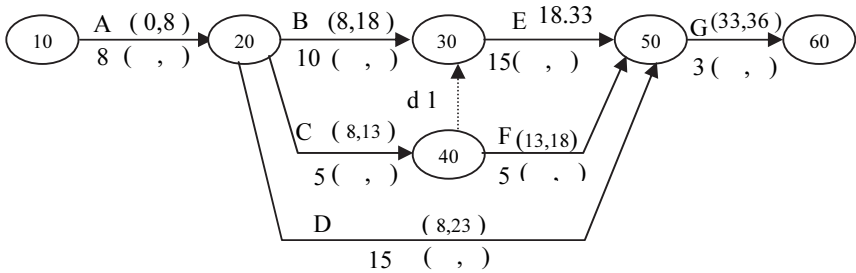
شكل (٦١-٣) حسابات الشبكة من اليسار إلى اليمين
