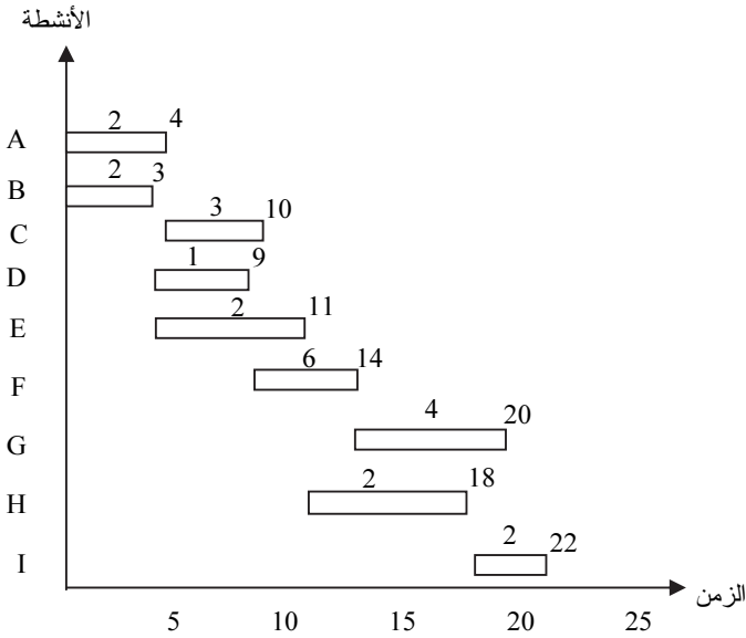
شكل (٣-٥) تمثيل البنود بطريقة الجدول البياني
