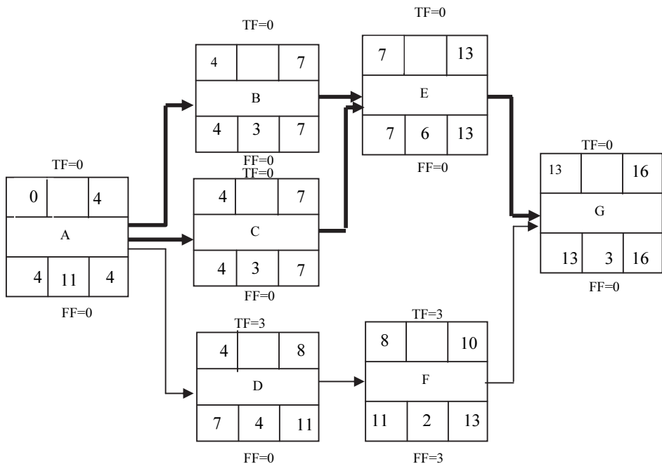
شكل (٣-٦٧) رسم وحساب الشبكة بطريقة المستطيلات
