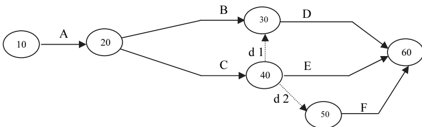
شكل (٣٠-٣) يمثل الشبكة بعد التجميع والترقيم
