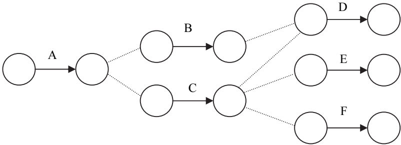
شكل (٣-٢٢) يمثل ربط الأنشطة مع بعضها البعض
