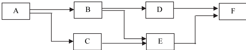
شكل (٣-٣٧) تمثيل الأنشطة بطريقة المستطيلات
