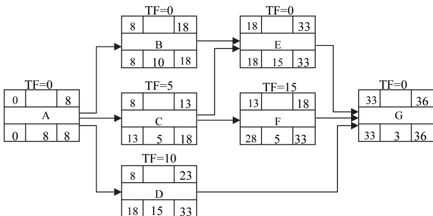
شكل (٣-٥٧) حساب فترة السماح الكلي (TF) لجميع الأنشطة
