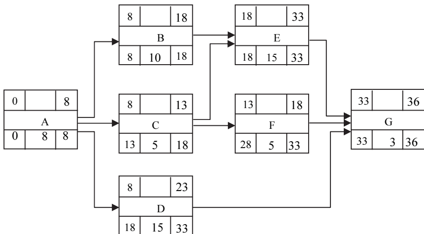
شكل (٣-٥٦) الشبكة في شكلها النهائي بعد تحديد البدايات والنهايات المبكرة والمتأخرة لجميع الأنشطة
