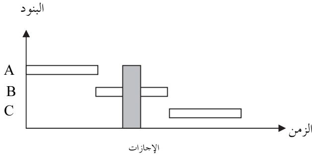
شكل (١-٣) تمثيل البنود بطريقة الجدول البياني (Bar chart)
