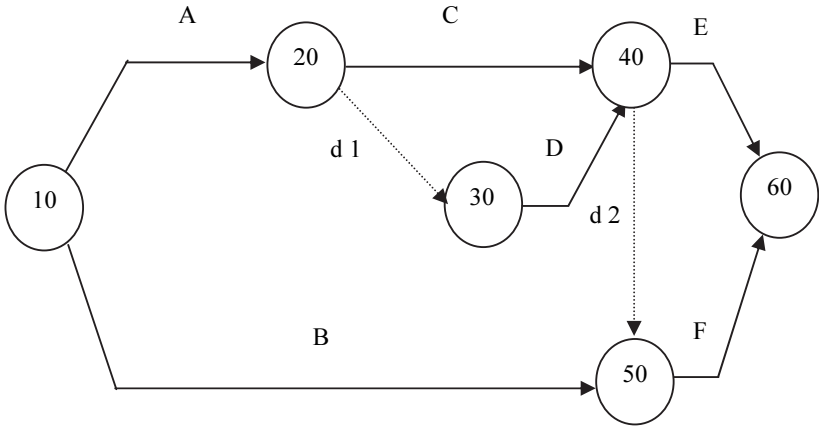
شكل (٣-٣٩) رسم الشبكة بطريقة الأسهم
