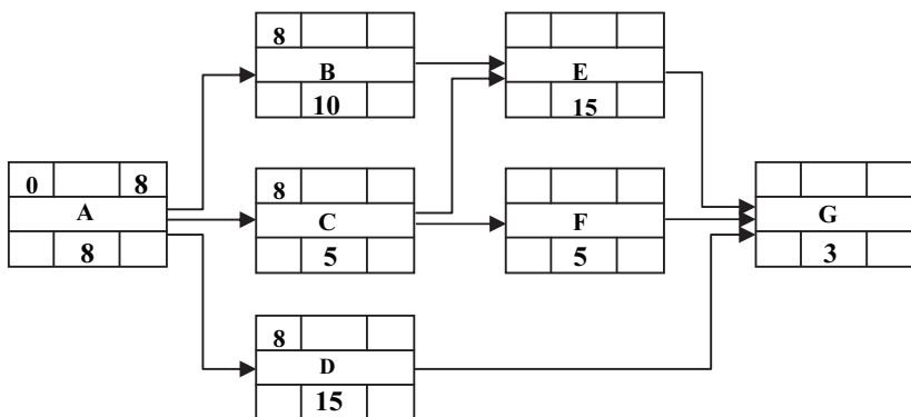
شكل (٣-٥٠) تحديد البدايات المبكرة للأنشطة (B&C&D)
