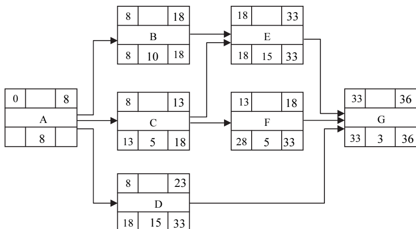
شكل (٣-٥٥) تحديد النهايات المتأخرة لكل من الأنشطة (B&C) وحساب البدايات المتأخرة لها
