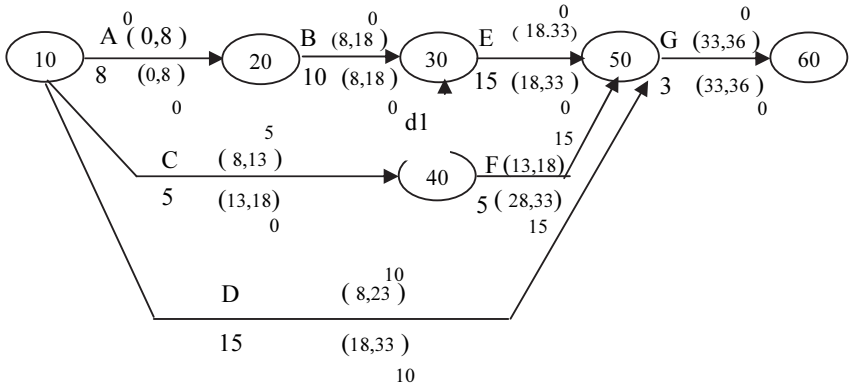
شكل (٣-٦٤) حسابات فترات السماح الحر للأنشطة
