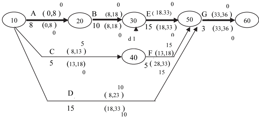
شكل (٣-٦٥) الشبكة النهائية مع تحديد المسار الحرج
