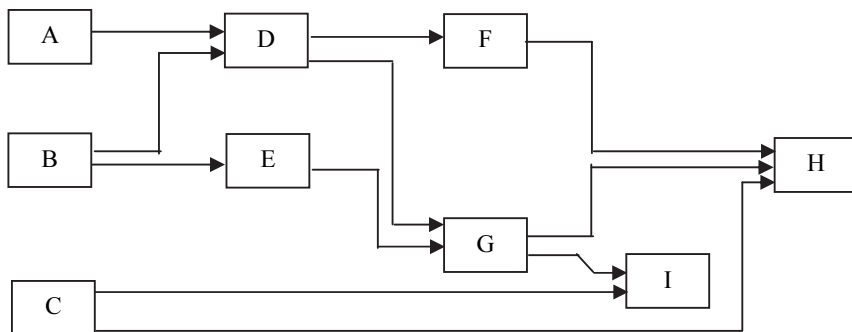
شكل (٣-٤٢) رسم الشبكة بطريقة الأسهم
