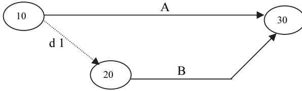
شكل (٣-١٧) إظهار الأنشطة الوهمية التي تعالج مشكلة التقييم
