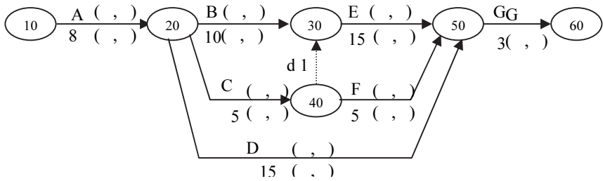
شكل (٦٠-٣) شبكة افتراضية لأحد المشروعات ممثلة بطريقة الأسهم
