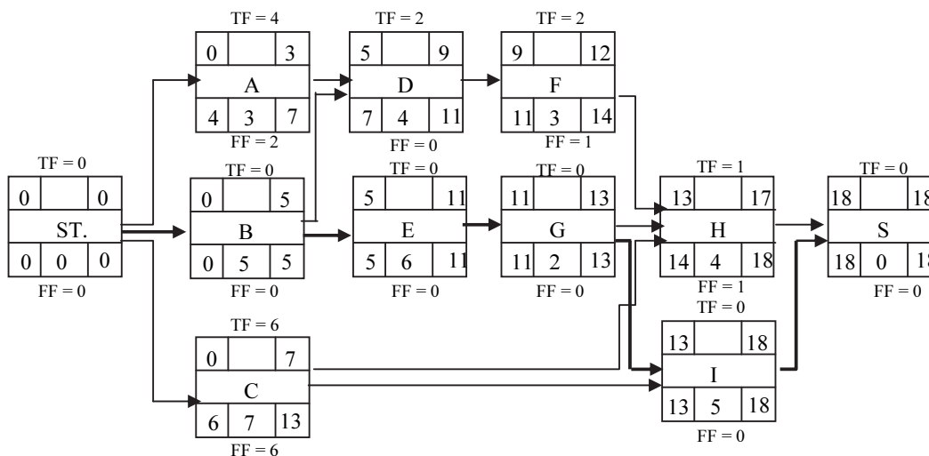
شكل (٣-٧١) رسم الشبكة بطريقة المستطيلات
