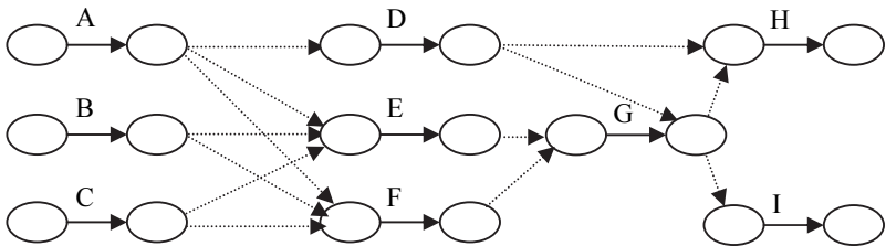
شكل (٣٢-٣) ربط الأنشطة طبقاً للعلاقات بينها
