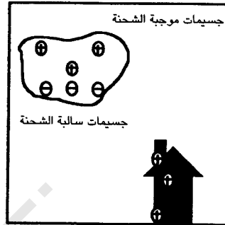
تسقط الجسيمات سالبة الشحنة إلى قعر السحابة
