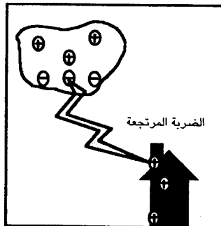
تندفع الجسيمات موجبة الشحنة من الأرض إلى الأعلى عبر نفس المسار
