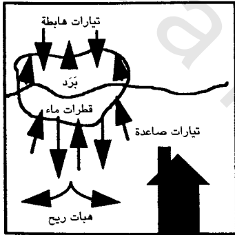
تقوم قطرات الماء وبلورات الثلج بجر الهواء إلى الأسفل
