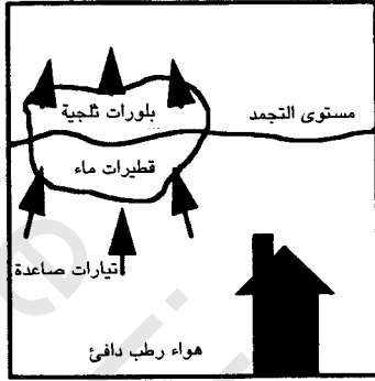
يرتفع الهواء الرطب الدافئ، يتكاثف بخار الماء مشكلاً سحابة
