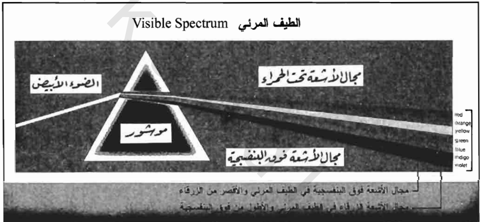
الحزم الضوئية للطيف المرئي
