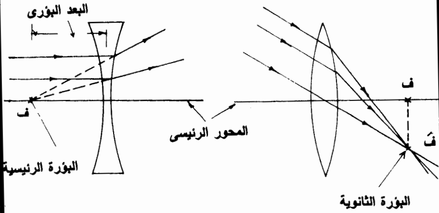
(ج) عدسة مقعرة (مشتتة)
