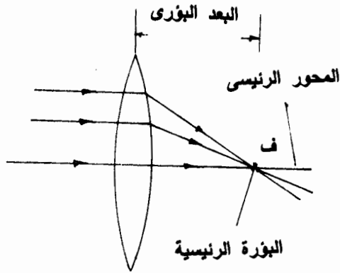
(أ) عدسة محدبة والأشعة موازية للمحور الرئيسي
