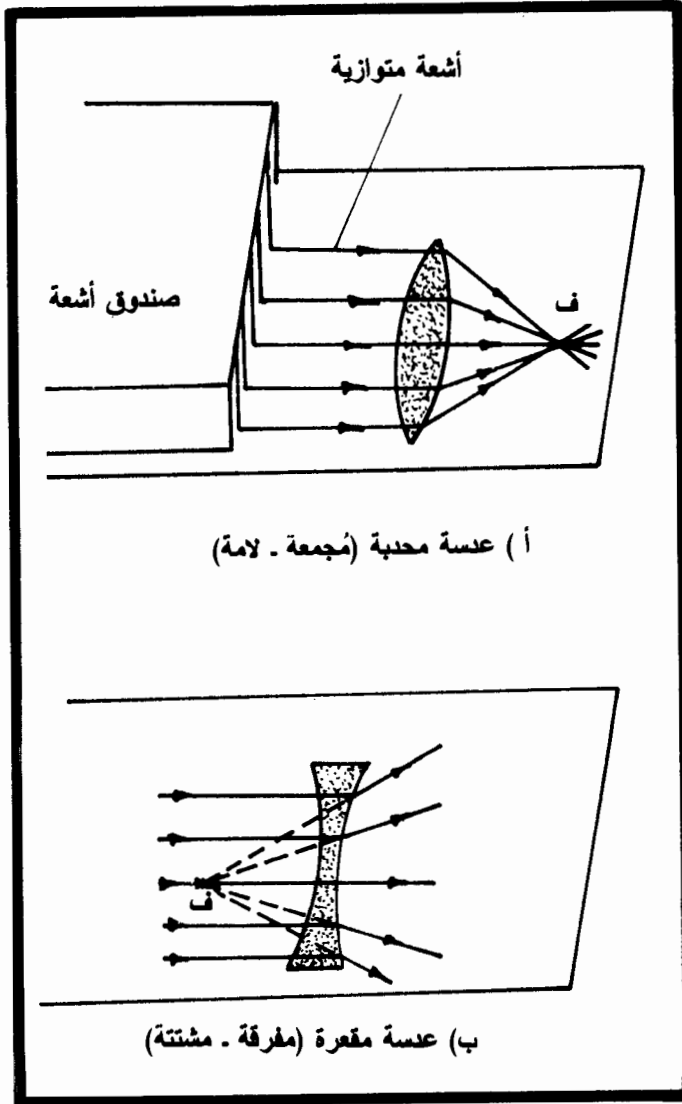
شكل [ ٤ - ١٣ ] الانكسار في العدسات المحدبة والمقعرة
