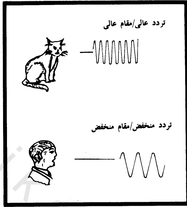
شكل [ ٢١ - ٤ ] يعتمد مقام الصوت على التردد
