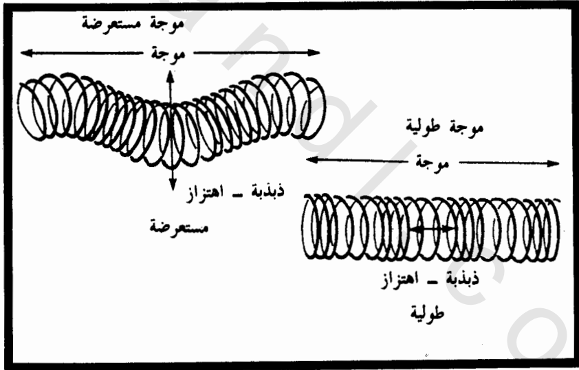
شكل [ ٢١ - ٢ ] الموجات المستعرضة والطولية
