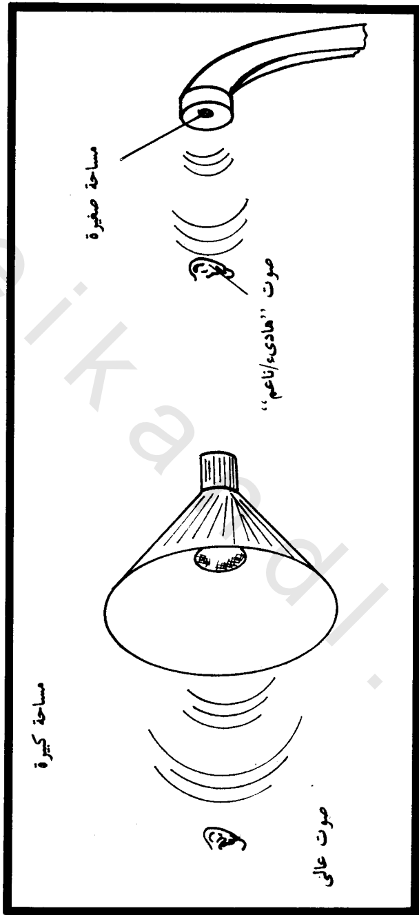
شكل [ ٦-١ ] الأصوات العالية والمنخفضة
