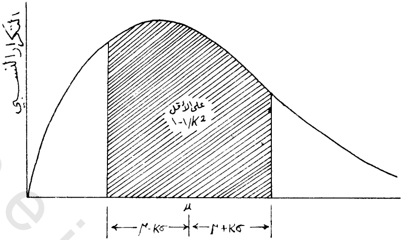
شكل ٢ - ٧ توضيح نظرية تشيبيشيف
