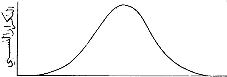
شكل ٢ - ٨ التوزيع الطبيعي
