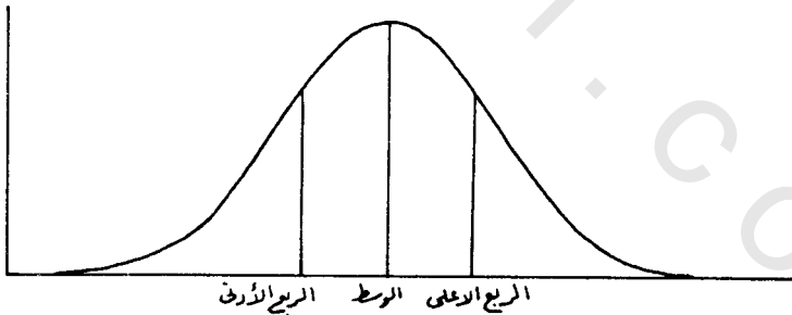
شكل (٢ - ٥) مواقع الأرباع
