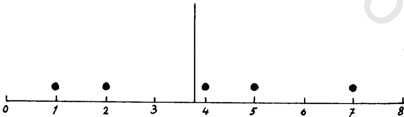
شكل (٢ - ٦) التمثيل البياني النقطي
